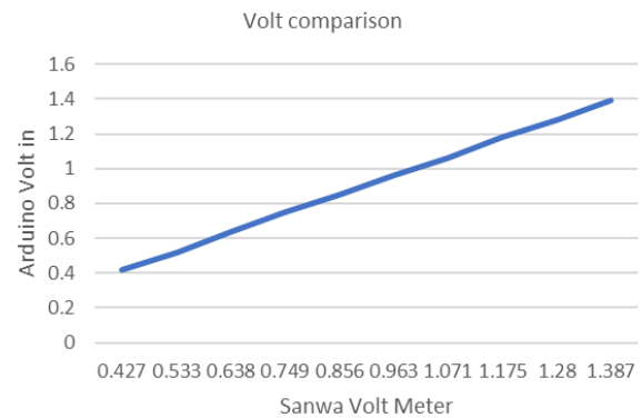
Fig. 11. Volt comparison
